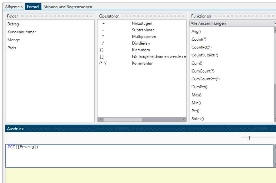
Abbildung 15-13: Einen neuen Ausdruck eingeben.
