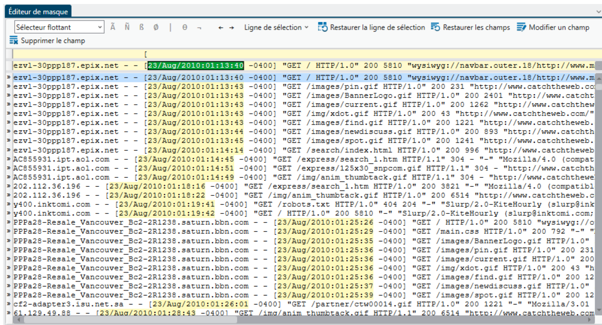
Figure 8-21. Prévisualisation du masque. Tous les champs de date/heure sont maintenant sélectionnés.
