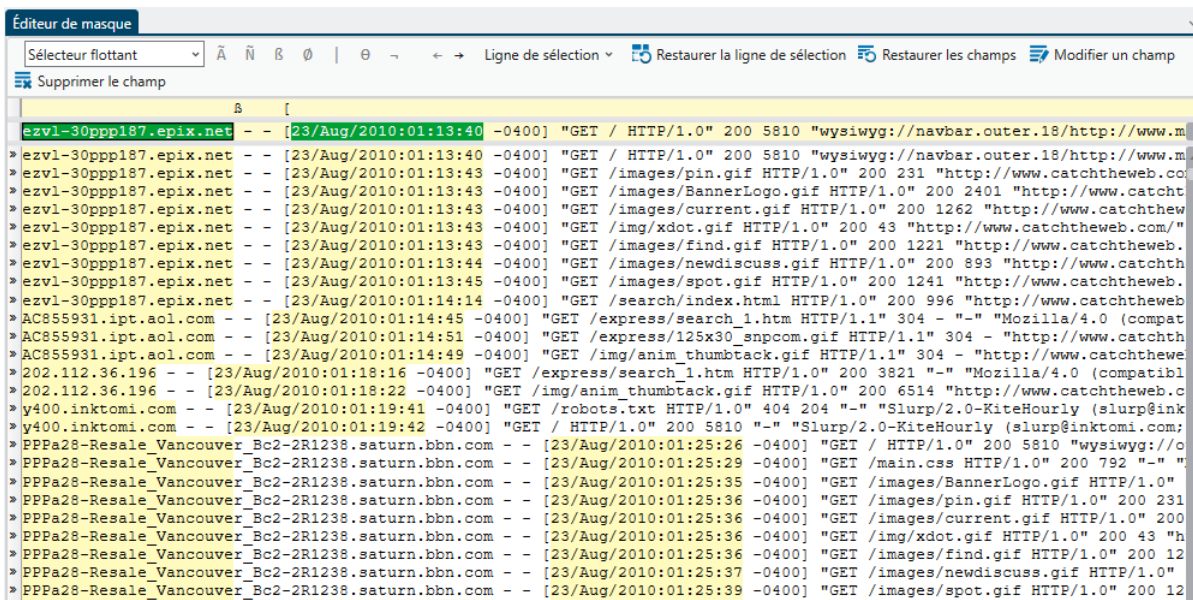
Figure 8-24. Sélecteur flottant avec champs de largeur variable.
