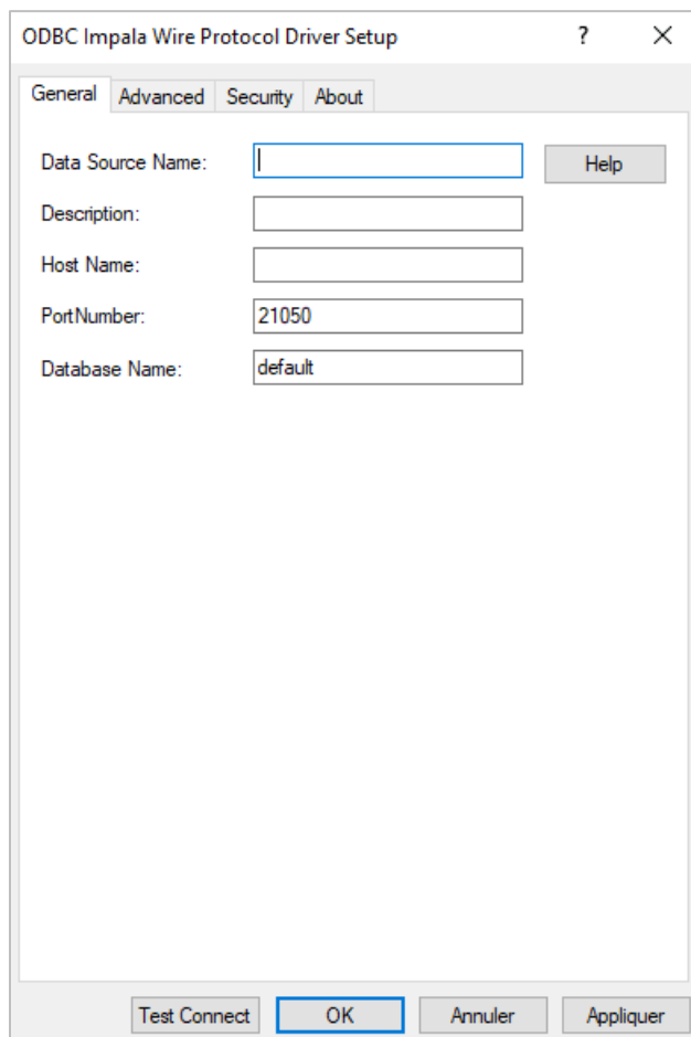
Figure 18-10. Boîte de dialogue de configuration du pilote ODBC Impala Wire Protocol.
