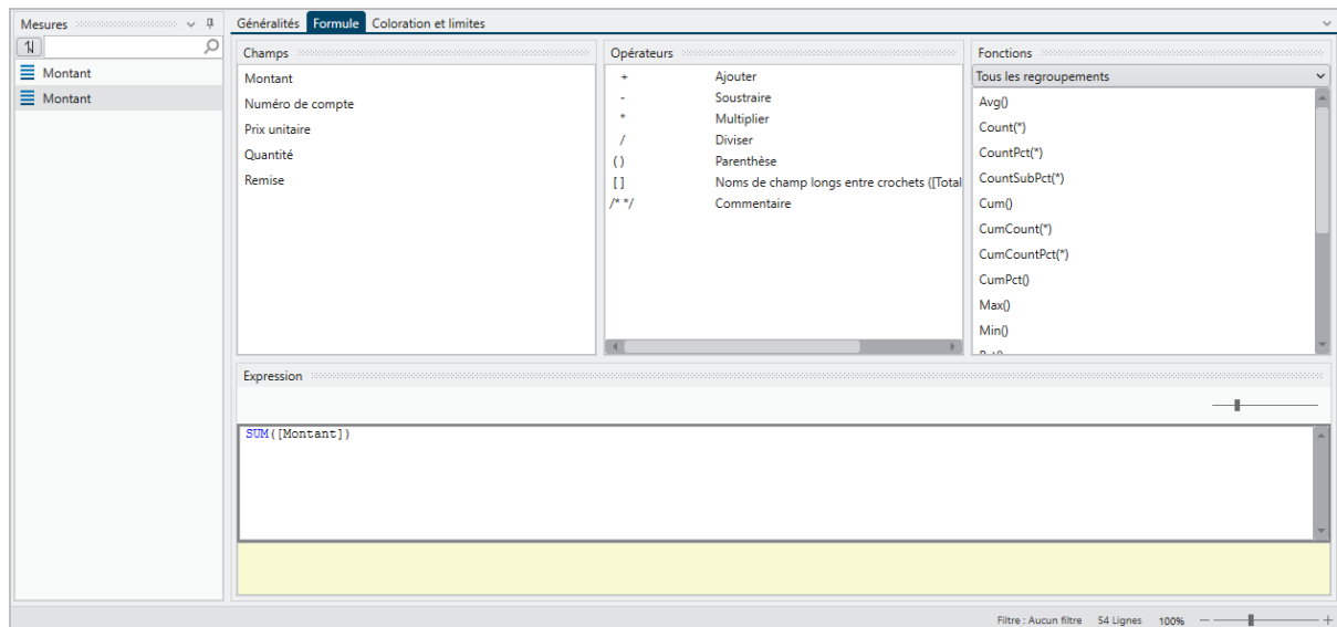
Figure 15-12. Options de Formule pour la nouvelle mesure Montant.
