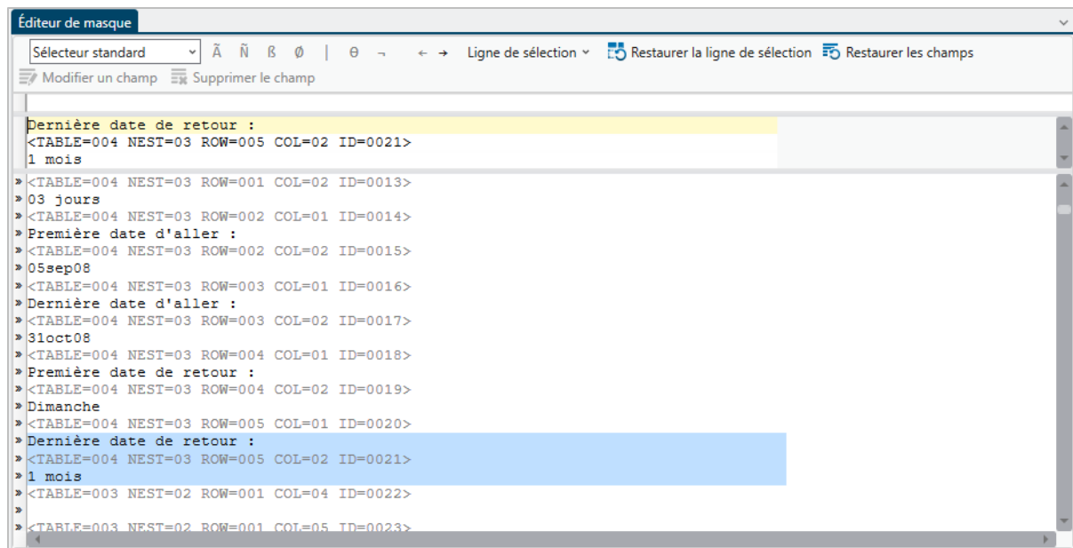
Figure 18-18. Sélection de l'information de « Dernière date de retour ».
