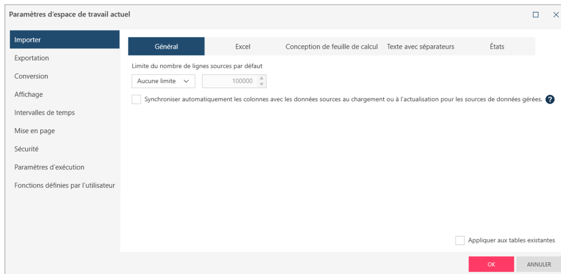
Figure 2-10. Boîte de dialogue Paramètres de l'espace de travail actuel de Data Prep Studio.
