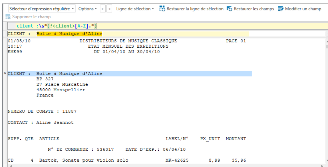
Figure 8-41. Création d'un sélecteur d'expression régulière.
