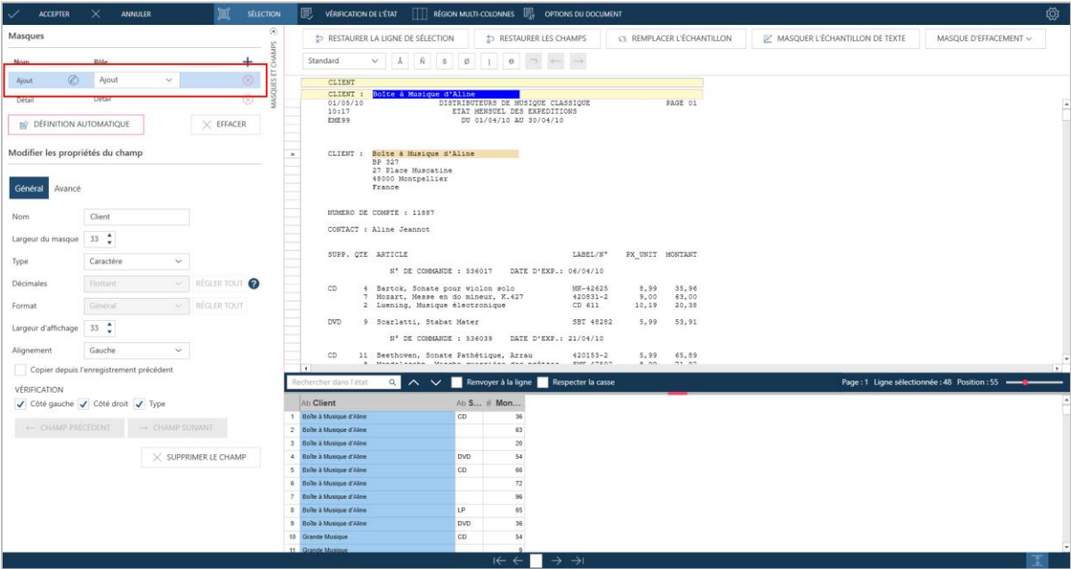
Figure 4-60. Extraction du champ Client de Classique.pdf depuis la fenêtre de conception de l'état
