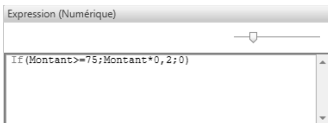
Figure 12-8. Définition modifiée du champ calculé Remise.
